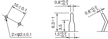
(基板孔尺寸)
