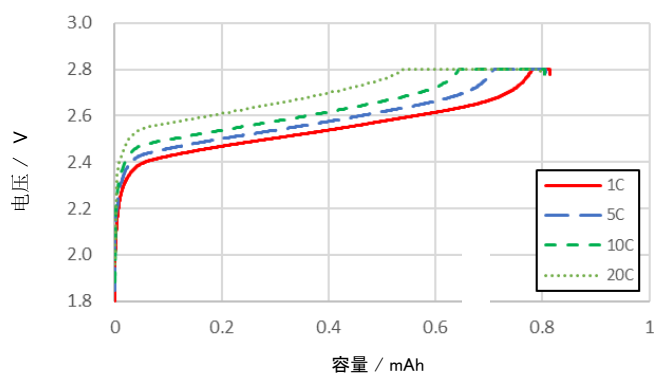
充电特性
