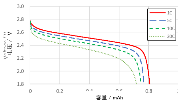
放电特性
