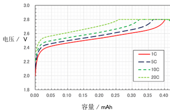
充电特性
