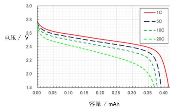
放电特性
